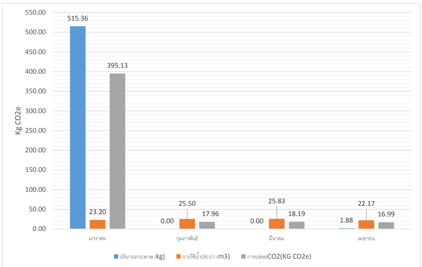
ภาพ 3 ปริมาณก๊าซเรือนกระจกทางอ้อมอื่น ๆ อาคารสำนักงานอธิการบดี เดือนมกราคม - เมษายน 2561
